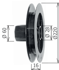
Puleggia AT222/22
