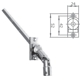
Snodo a piastra stretta
