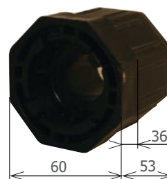
Calotta AT284 Ø 40
