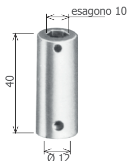
Boccola di collegamento fra argani
